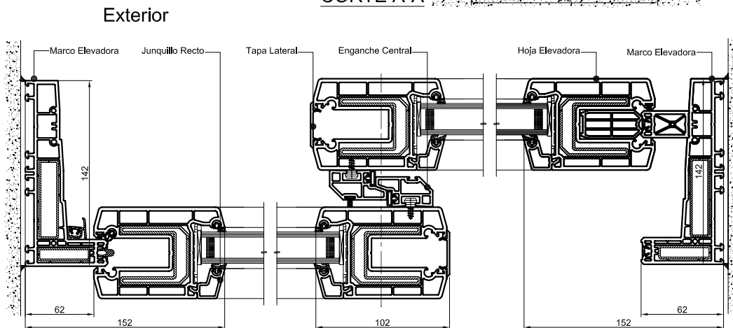
CORTE A-A
